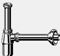
Pungvattenlås - förkromad mässing Tillbehör Kopp Ø 50 mm, rosett Ø32xØ80xH24 mm kvalitetskontroll enligt DIN EN 274 Modell 5753.905
