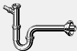
Rörvattenlås Plus siphon - förkromad mässing Tillbehör Skruvkoppling G 3/4, låsplatta, avsticksrör 200 mm, utloppsböj 220 mm Kvalitetskontroll enligt DIN EN 274 Modell 5611.6
