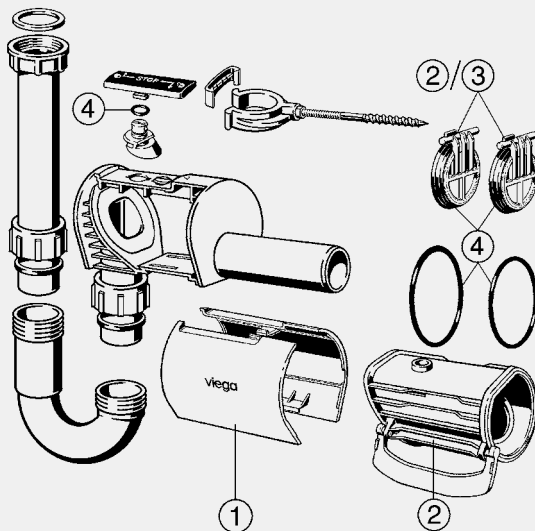
Sperrfix tättningsslack - avsedd för Sperrfix backventil typ 5 modell 4995.1 - bild 1 Modell 4995.95
