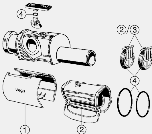
Sperrfix tätningslock - avsedd för Sperrfix backventil typ 2 modell 4995.3 - bild 1 Modell 4995.91
