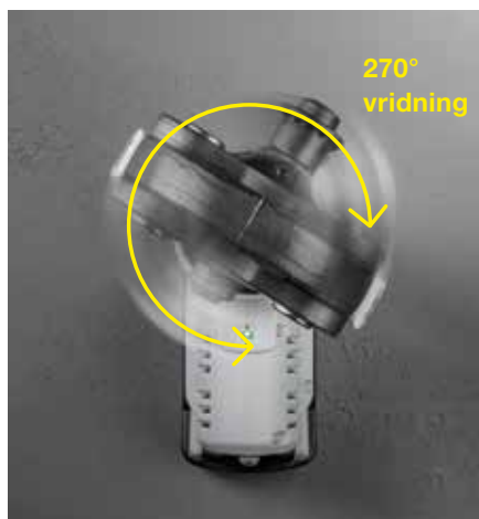
Pressbackfixturen, som är vridbar 270°, underlättar arbetet på svåråtkomliga ställen.
